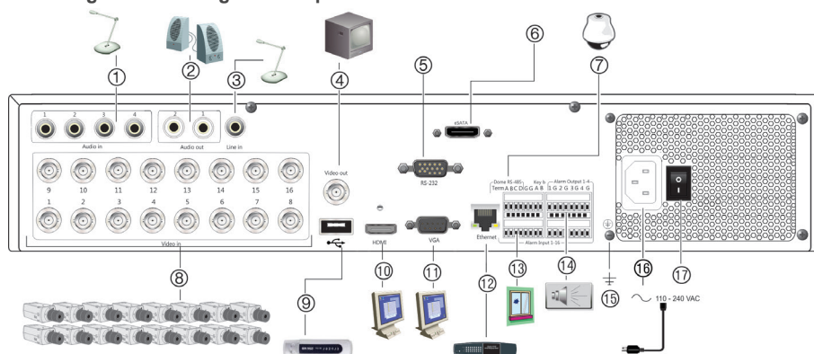
Afbeelding 1: Aansluitingen achterpaneel
